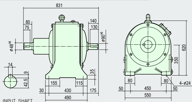
INPUT SHAFT
