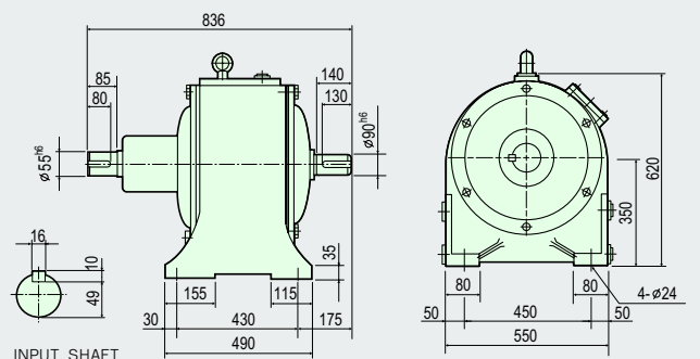
INPUT SHAFT
