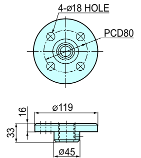
플랜지 너트 Flange Nut
