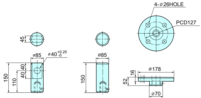
크레비스 너트 Clevis Nut
