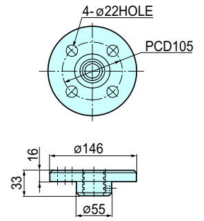
플렌지 너트 Flange Nut
