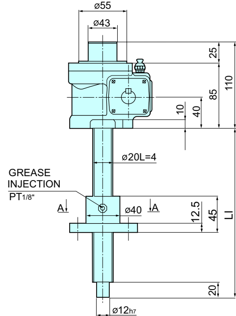
하방향형 Inverted Traveling
