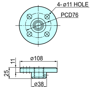
플랜지 너트 Flange Nut
