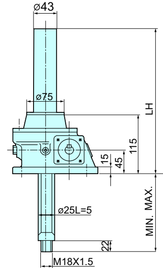
하방향형 Inverted Traveling
